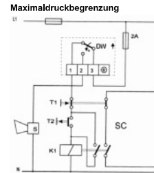
Abb. 6. Maximaldruckbegrenzung DW = Druckschalter T1 = STOP T2 = START
