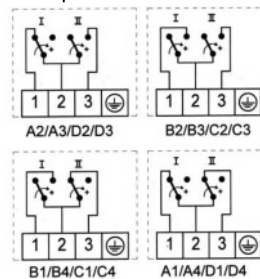
Abb. 15. Anschlußpläne ...-217 Bitte unbedingt Aufkleber neben dem Steckanschluß am Druckschalter beachten.
