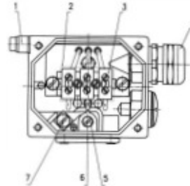
Fig. 21. Schaltpunkteinstellung
