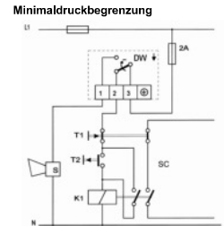
Abb. 7. Minimaldruckbegrenzung S = Signal (nach Bedarf) K1 = Relais mit Selbsthaltung SC = Sicherheitsstromkreis
