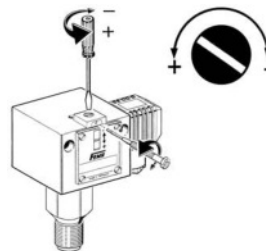
Abb. 5. Einstellen des Schaltdrucks
