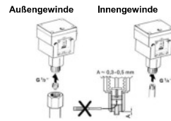
Abb. 3. Druckschalter
