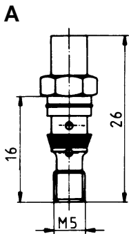
Drehspindel mit Schlitzschraube versenkt Spindle with slotted screw sunk-in
