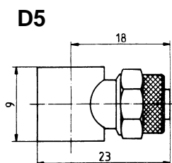
Rapidverschraubung Rapid fitting
