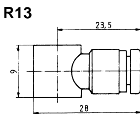
Steckverschraubung Push-in fitting
