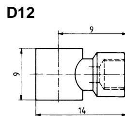
Verschraubung mit IG Fitting with female thread
